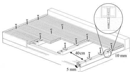
Zdjęcie poglądowe - montaż na klipsy
